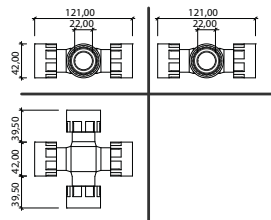
CROSS FxFxFxF 1"
